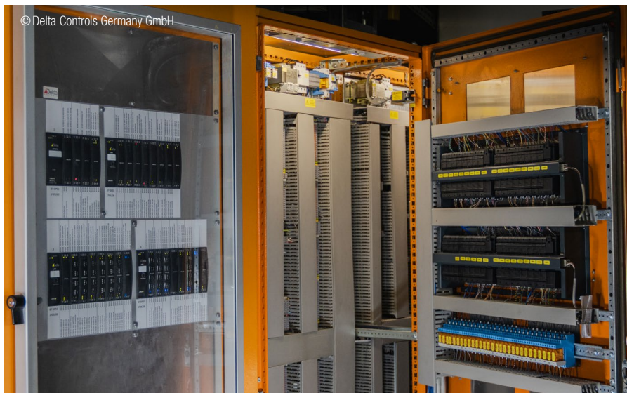
Gebäudeautomatonschaltschrank im Keller der Gebäude am Potsdamer Platz. Building automation control cabinet in the basement of the buildings at Potsdamer Platz.
