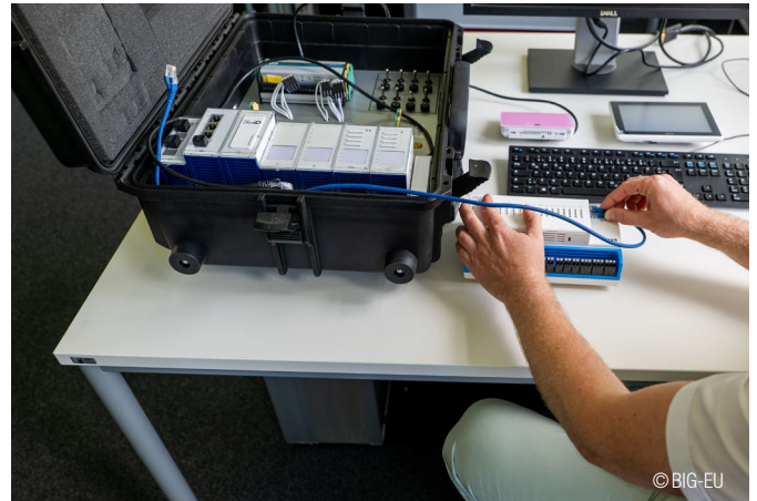
Anschluss eines TP-Kabels zur Datenübertragung im Labor der FH Aachen. Connection of a TP cable for data transmission in the FH Aachen laboratory.
